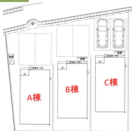
配置図
